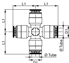
croix égale
