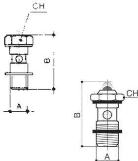
rondelles-joints montées
